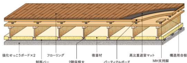
三井ホームの開発した高遮音床「MOCX MUTE（モクスミュート）」。 本技術では床根太部分が CLT となります。
